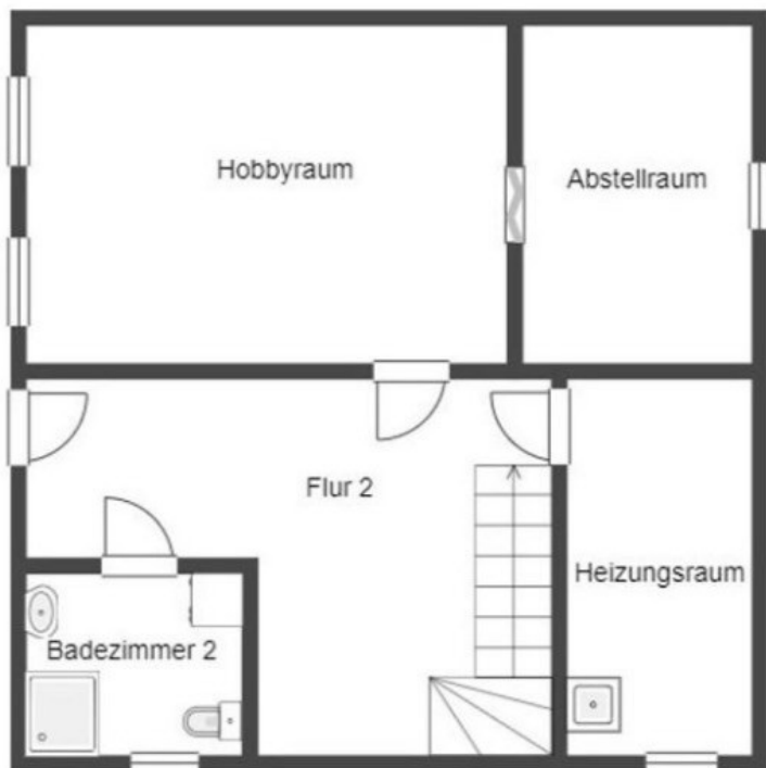
Grundriss Skizze UG
